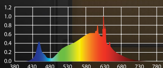
Réglage de luminaire 3000K avec optique claire standard
