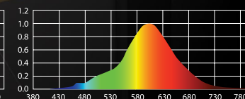
Réglage de luminaire 3000K avec optique ambre = 2200K CCT
